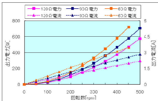
図 2 回転数 - 出力特性
