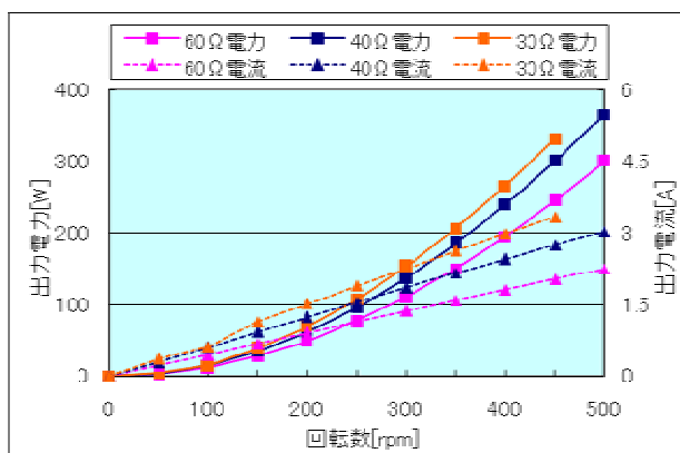
図 2 回転数 - 出力特性
